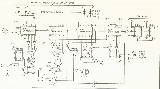
Fig. 31-24. Programmable divider ( \div N ).
